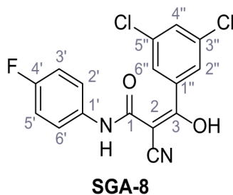
Chemical structure 49. Cyano-3-(3,5-dichlorophenyl)-N-(4-fluorophenyl)-3-hydroxyacrylamide – SGA-8.
