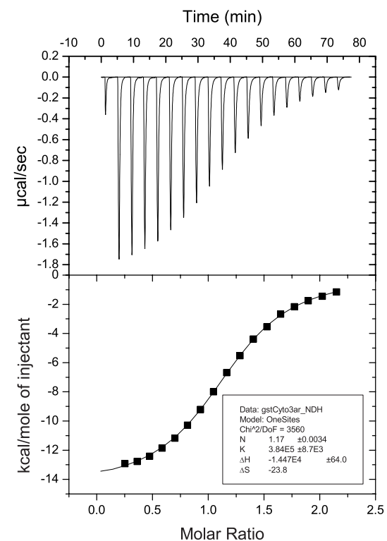
30 μM GST-CNNM3 299-658 300 μM ARL15 32-197
