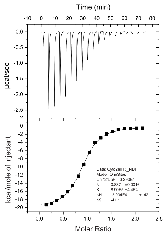
30 μM CNNM2 429-817 300 μM ARL15 32-197
