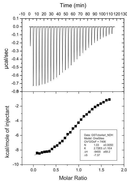
30 μM GST-CNNM4 356-511 300 μM ARL15 32-197
