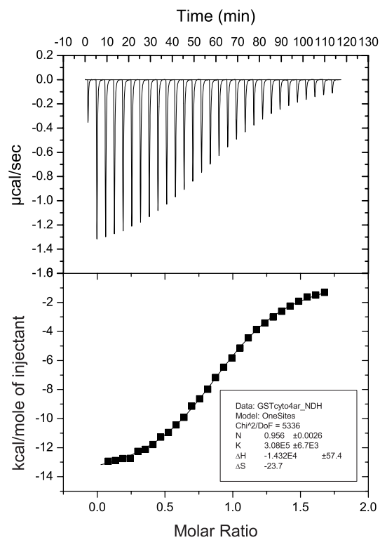
30 μM GST-CNNM4 356-726 300 μM ARL15 32-197
