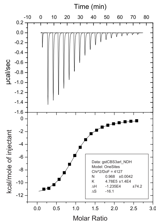
30 μM GST-CNNM3 299-452 300 μM ARL15 32-197
