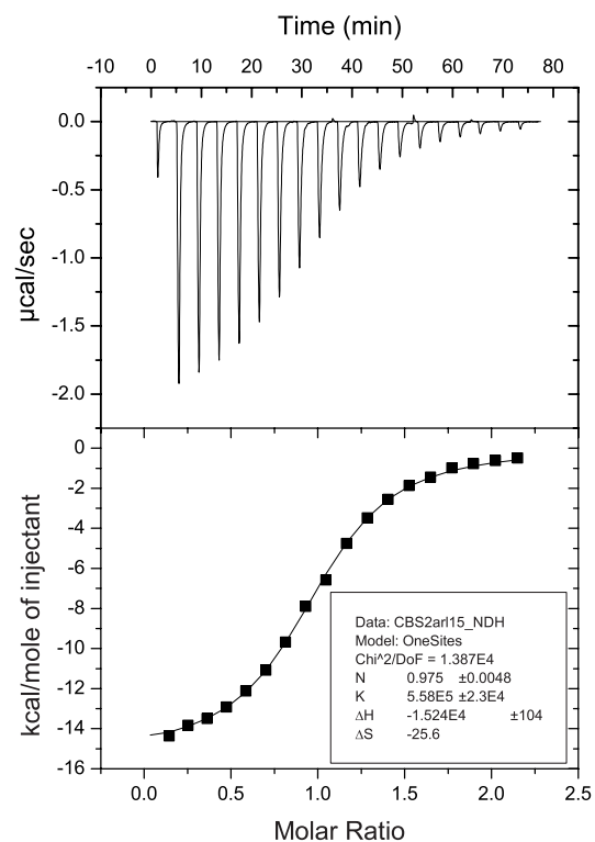
30 μM CNNM2 429-584 300 μM ARL15 32-197
