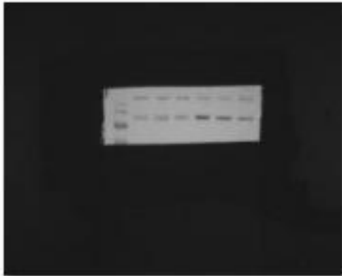
P-HSF1 (Ser 320)
