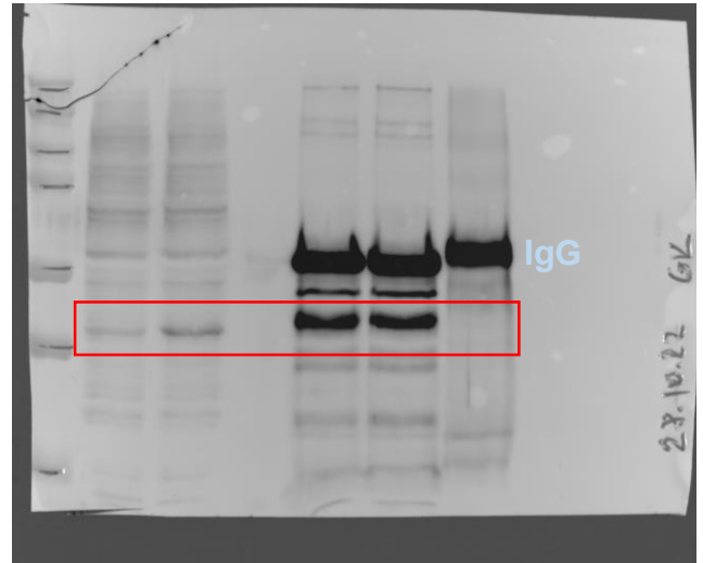
L1 ORF1p
